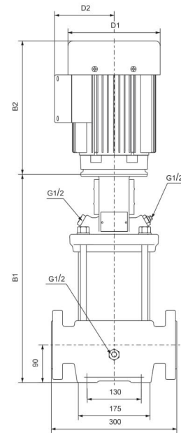
DIN FLANGE(LVR)/F
