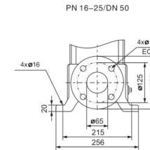
DIN FLANGE(LVR)/F
