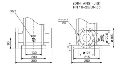
DIN FLANGE(LVS)/F
